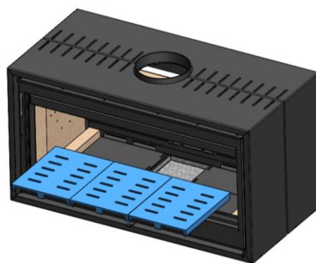
Figura n°20 - Extraemos las parrillas de fundición.
