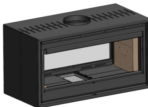
Figura n°21 - Extraer el refractario inferior restante del lado derecho.
